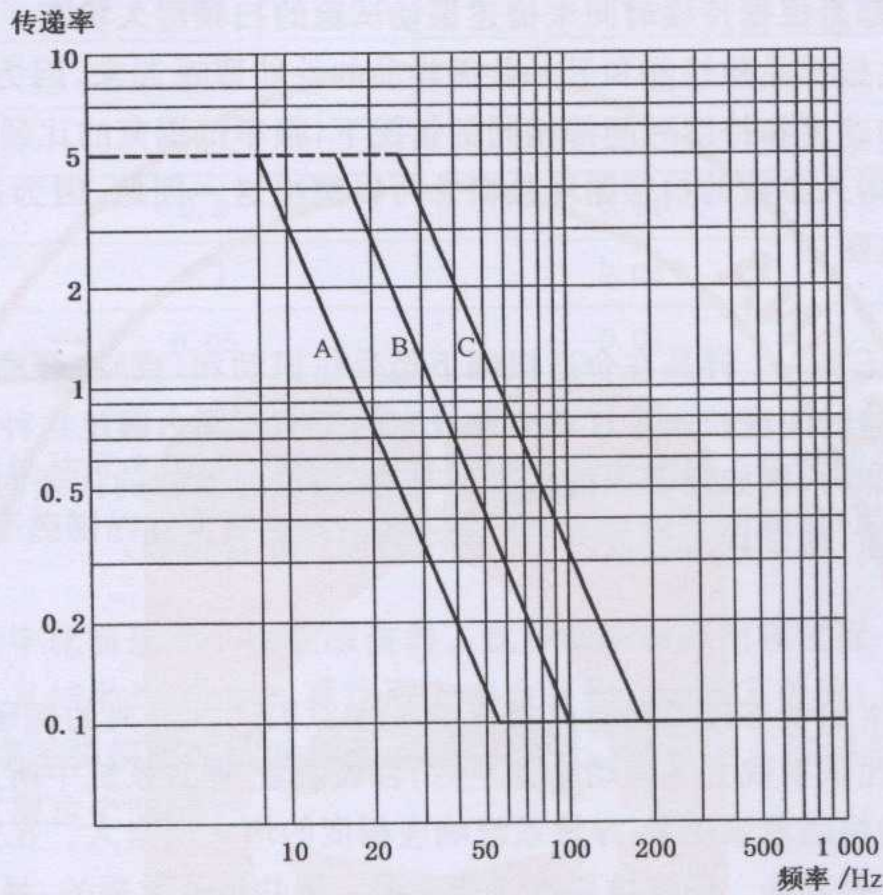
图 A.1 减振器的一般传递特性曲线
